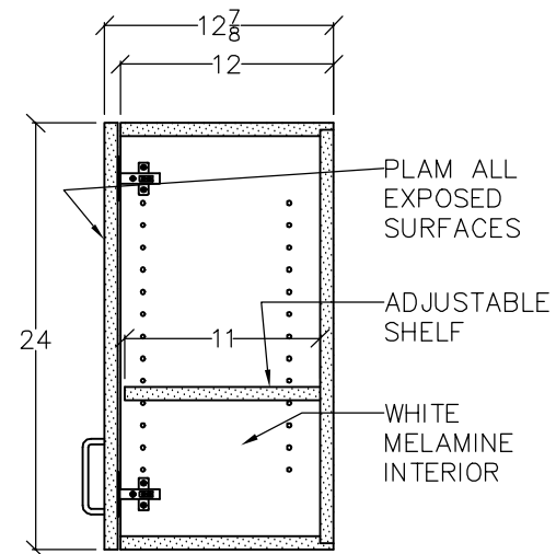
E 24" WALL CABINET SCALE: 1" = 1'
