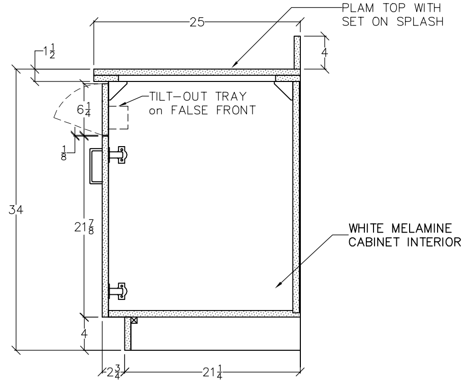
B SINK BASE SCALE: 1" = 1'
