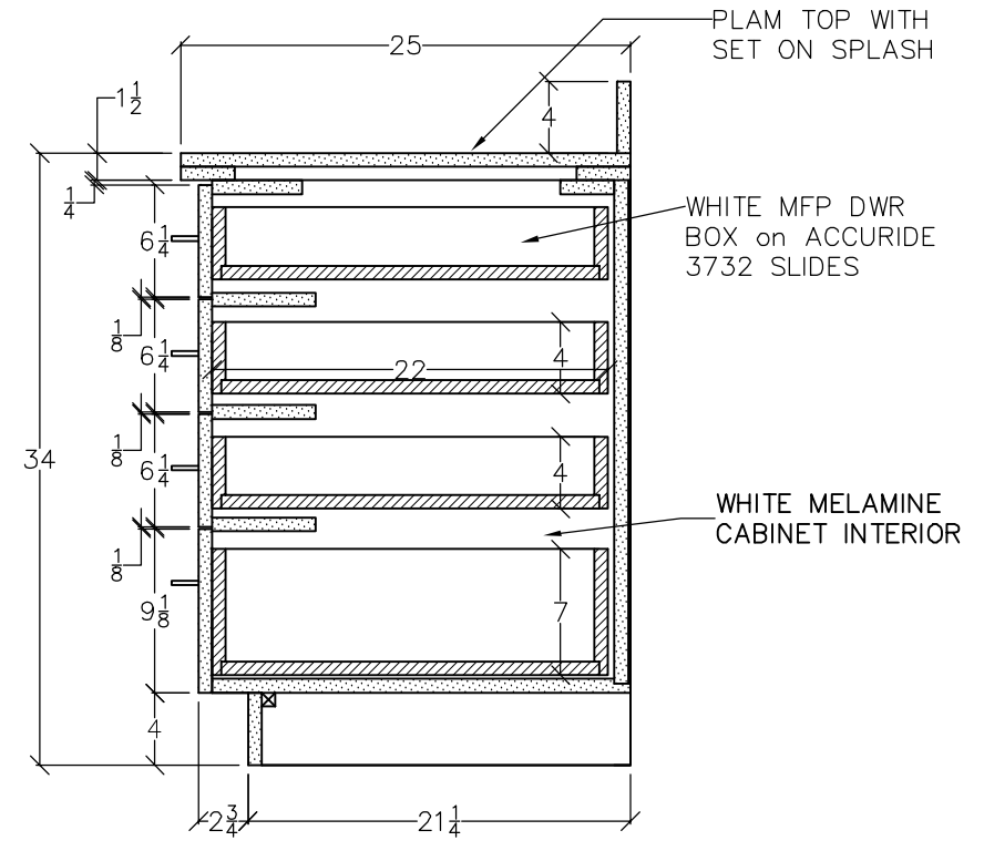
C BASE CABINET SCALE: 1" = 1'
