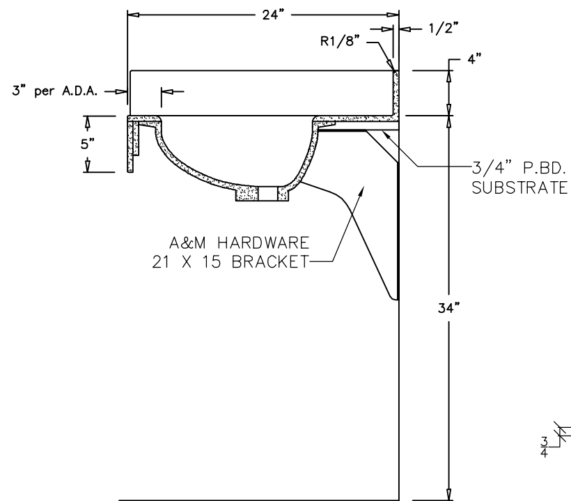
R BASE CABINET SCALE: 1" = 1'
