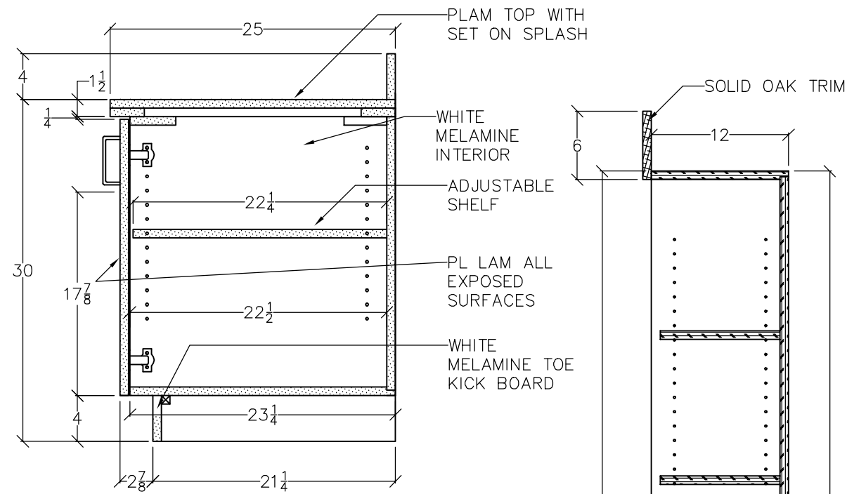
R BASE CABINET SCALE: 1" = 1'
