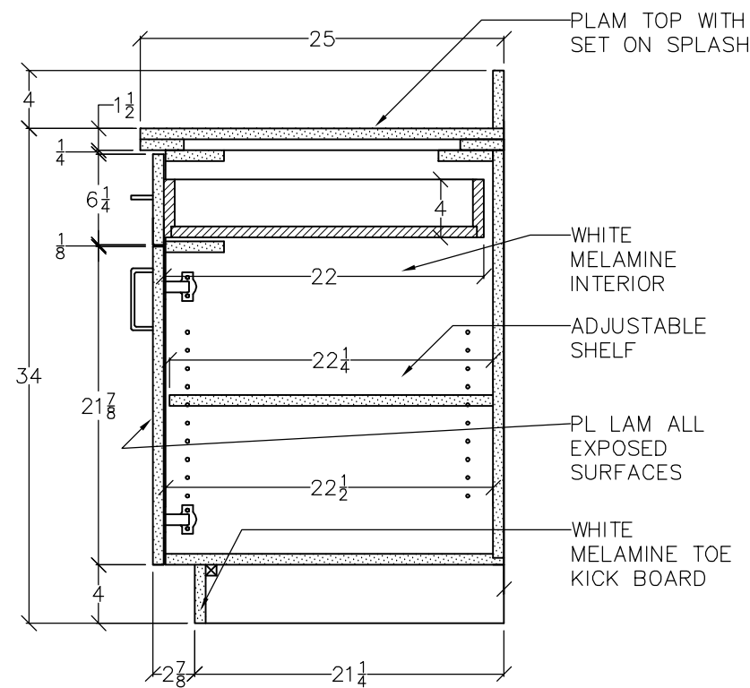
A BASE CABINET SCALE: 1" = 1'
