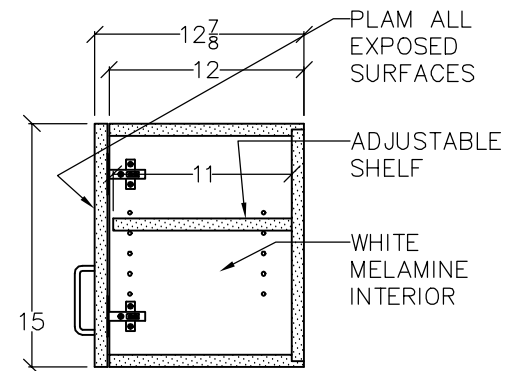
F 15" WALL CABINET SCALE: 1" = 1'
