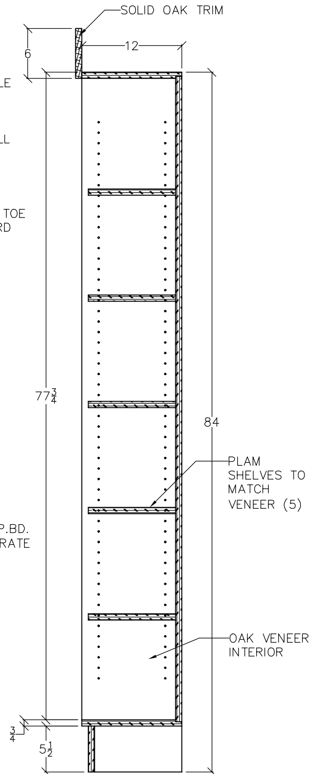
V BOOKCASE DETAIL SCALE: 1" = 1'
