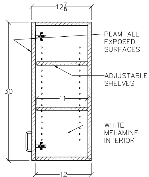
D 30" WALL CABINET SCALE: 1" = 1'
