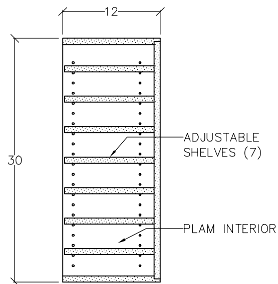
X 30" MAIL SORTING CAB SCALE: 1" = 1'
