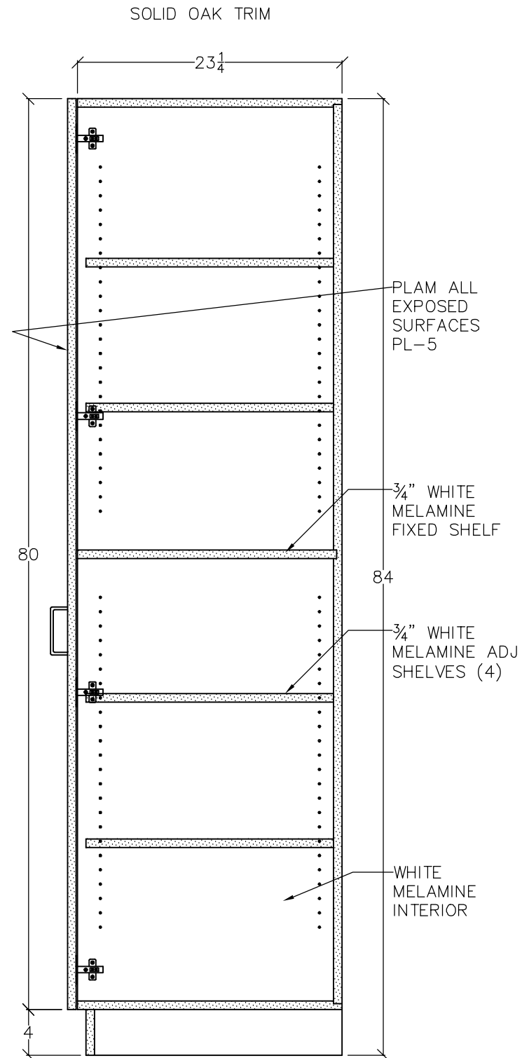
Y TALL CABINET SCALE: 1" = 1'
